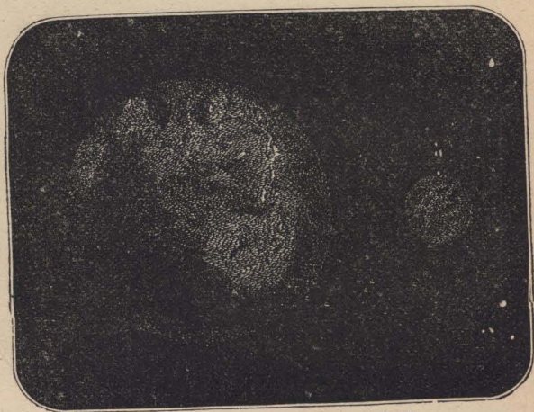
Tamaños comparados de Neptuno y de la Tierra.
